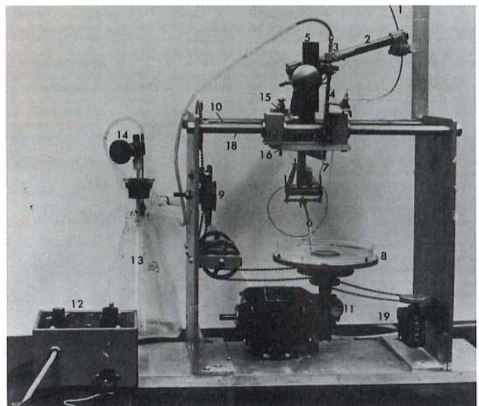
Bild 4 Der von J.E. Gilchrist und Kollegen entwickelte Prototyp Spiralplattierer
