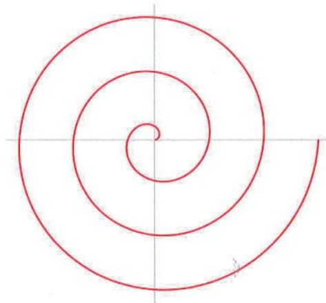
Bild 2 Archimedische Spirale nach f: \rightarrow (r\cos\delta, r\sin\delta) = (a\delta\cos\delta, a\delta\sin\delta)
